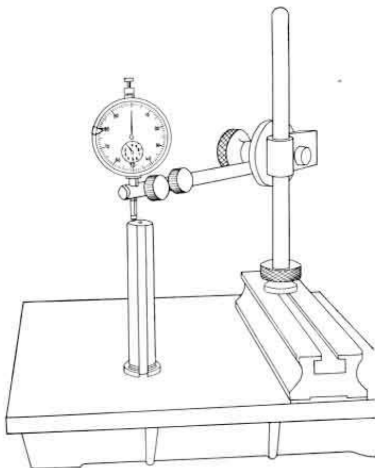
Fig. 18. - Azzeramento del comparatore sull'attrezzo A. 70037.
