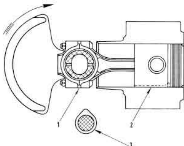
Fig. 7. - Mod. 500 Giardiniera - Schema per il montaggio del complessivo biella-stantuffo sul motore.
