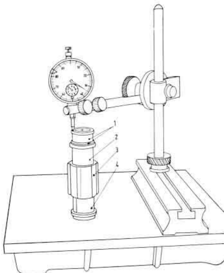
Fig. 19. - Lettura del valore « c » sul comparatore.
