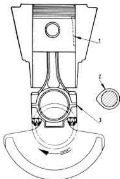
Fig. 6. - Modd. 500 L - 500 - 500 D e Nuova 500 Sport - Schema per il montaggio del complessivo biella-stantuffo sui motori. 1. Taglio di dilatazione - 2. Albero distribuzione - 3. Numerazione della biella.
